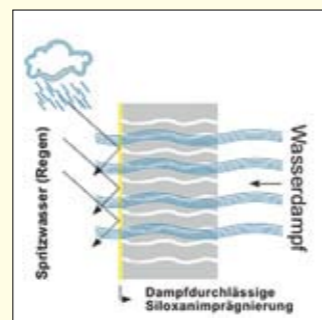
Mit Polysiloxan bzw. Hydrophob FAC behandeltes Mauerwerk.
